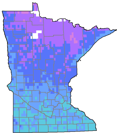
PCM B1
